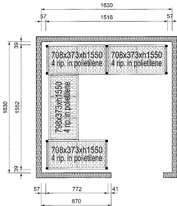
Boven aanzicht
